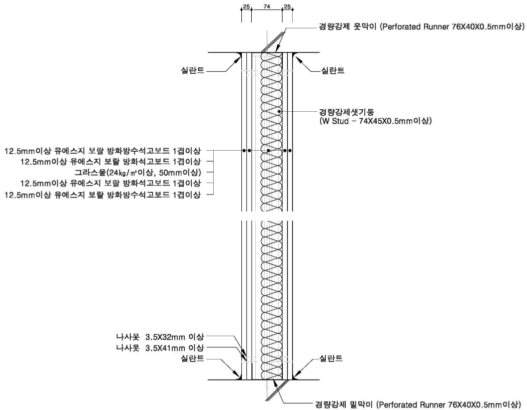
<수직단면도>
