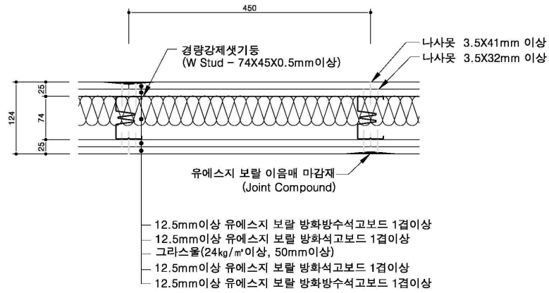
<수평단면도>
