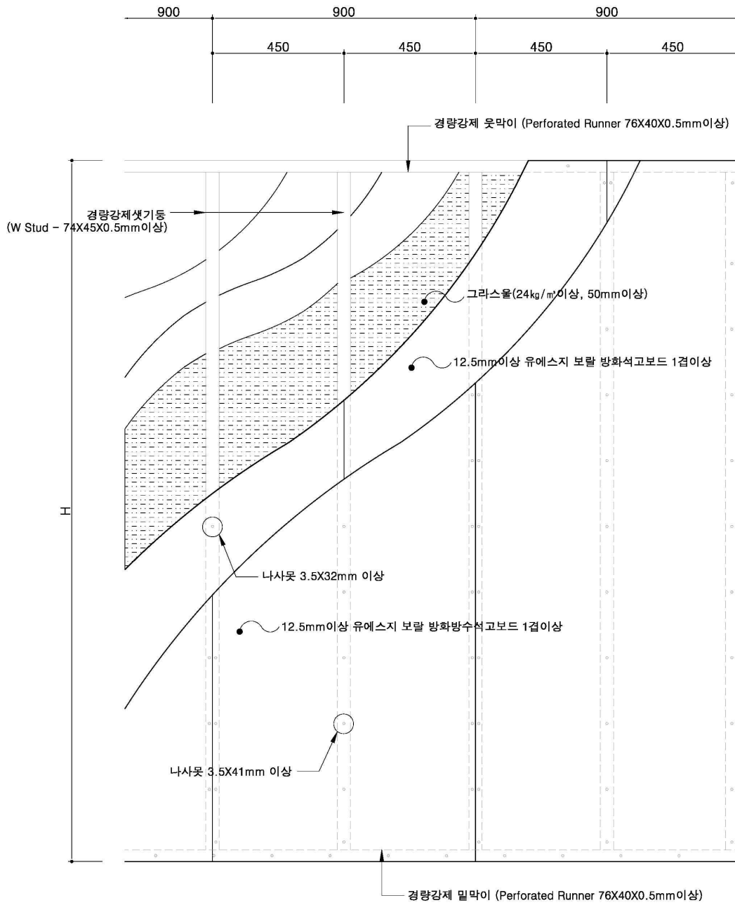
<입면도>
