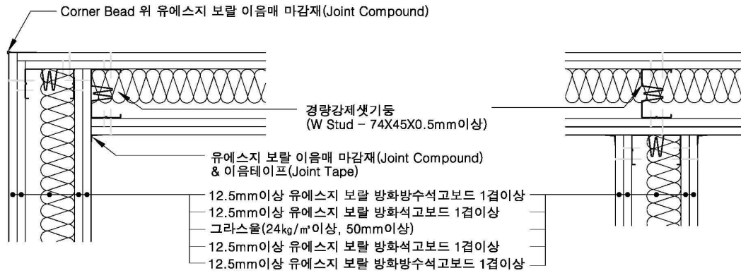
[ “┌” 접합부위 상세도 ]
