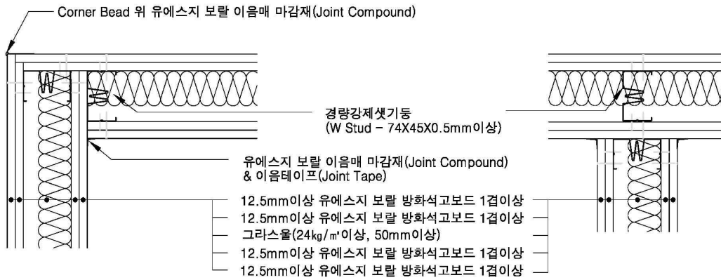
[ “ㄱ” 접합부위 상세도 ]
