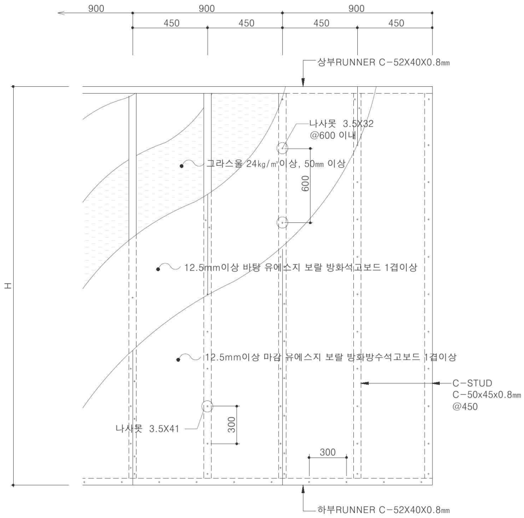
<입면도>
