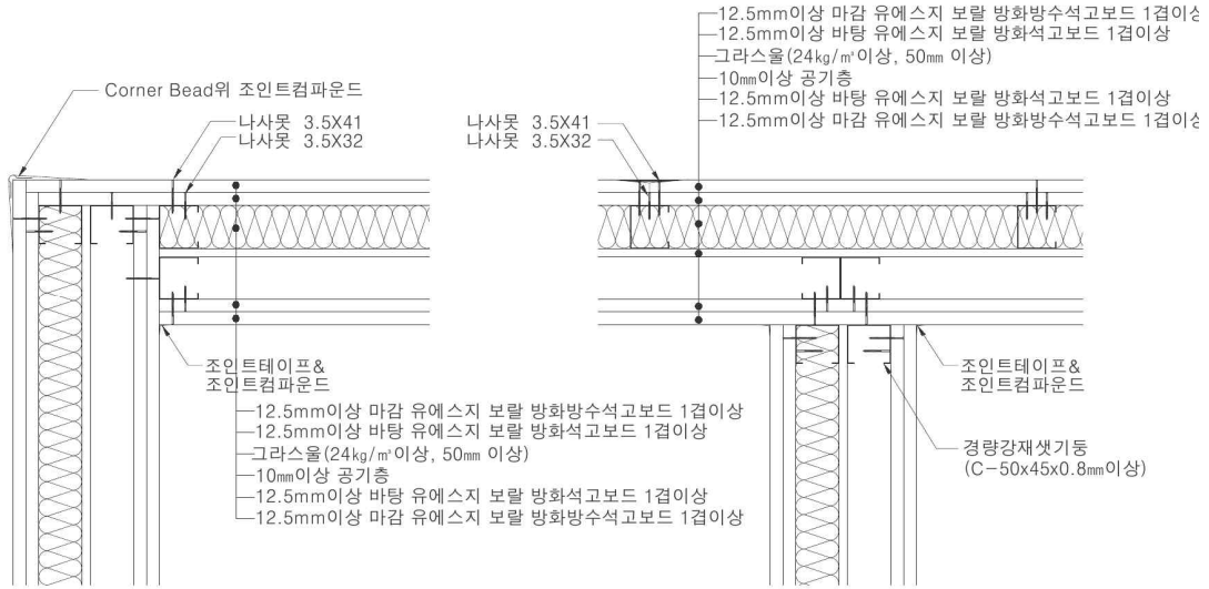
[ “ㄱ” 접합부위 상세도 ]
