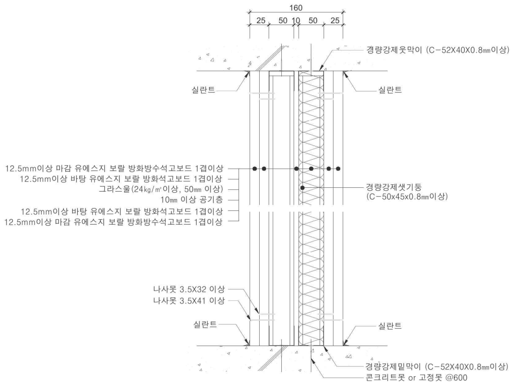
<수직단면도>
