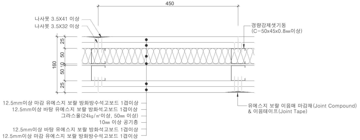
<수평단면도>
