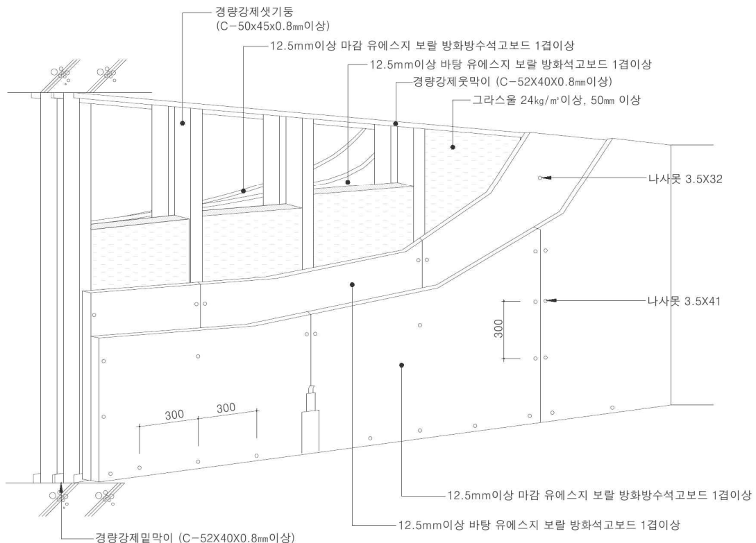
<투시도>
