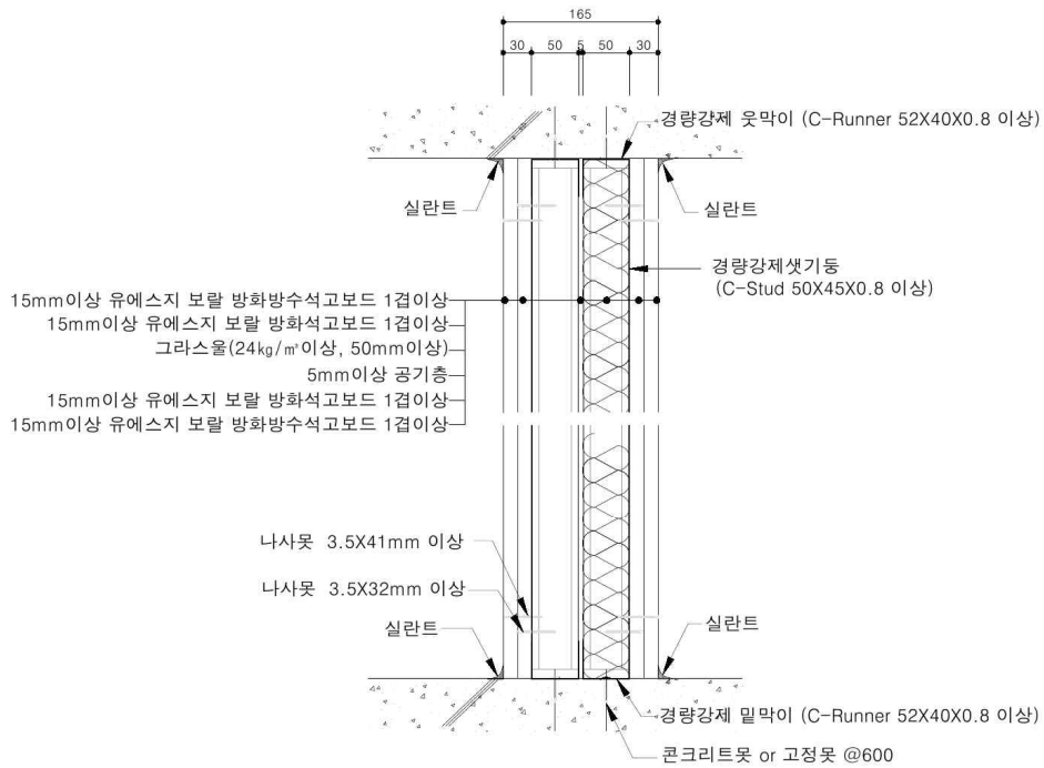
<수직단면도>
