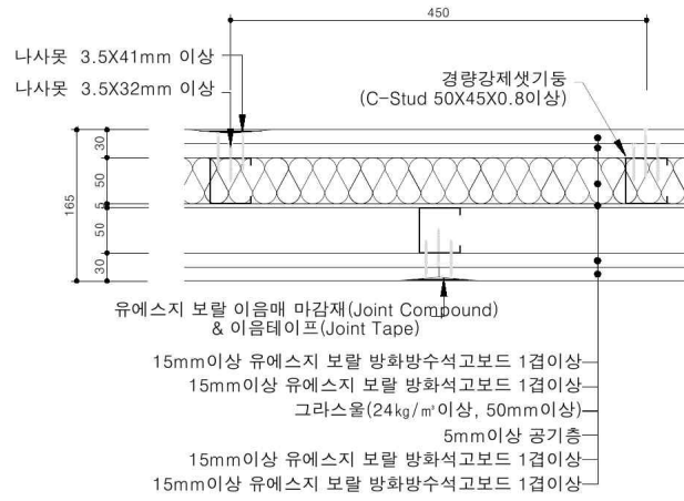
<수평단면도>
