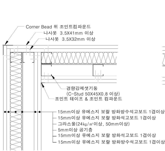
[ “┌” 접합부위 상세도 ]
