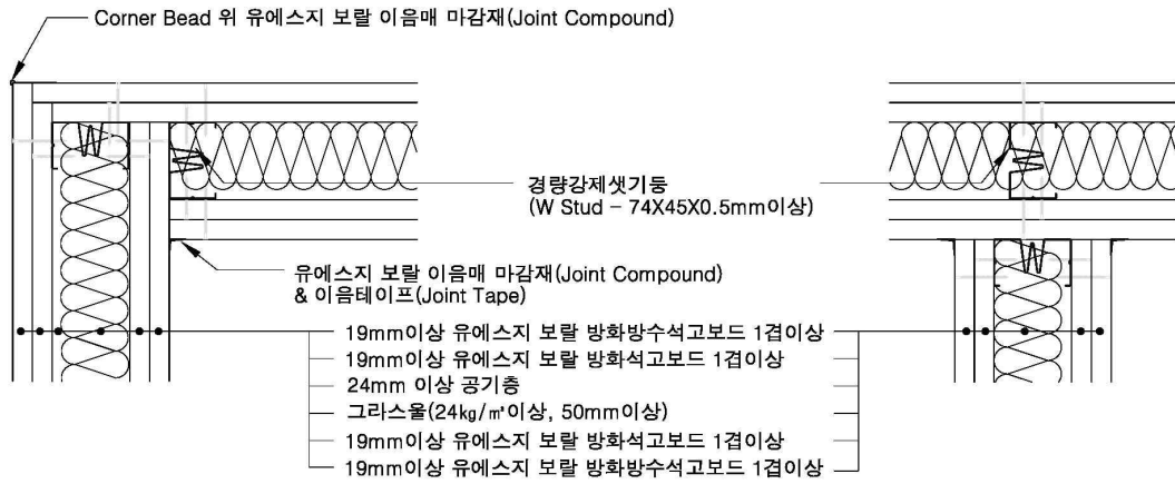
[ “ㄱ” 접합부위 상세도 ]
