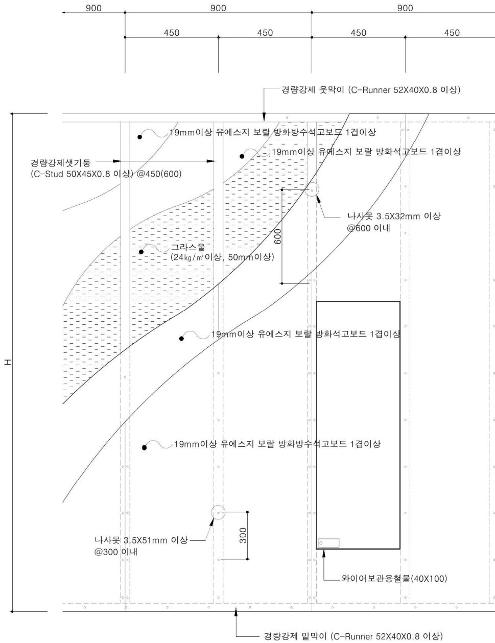
<입면도>
