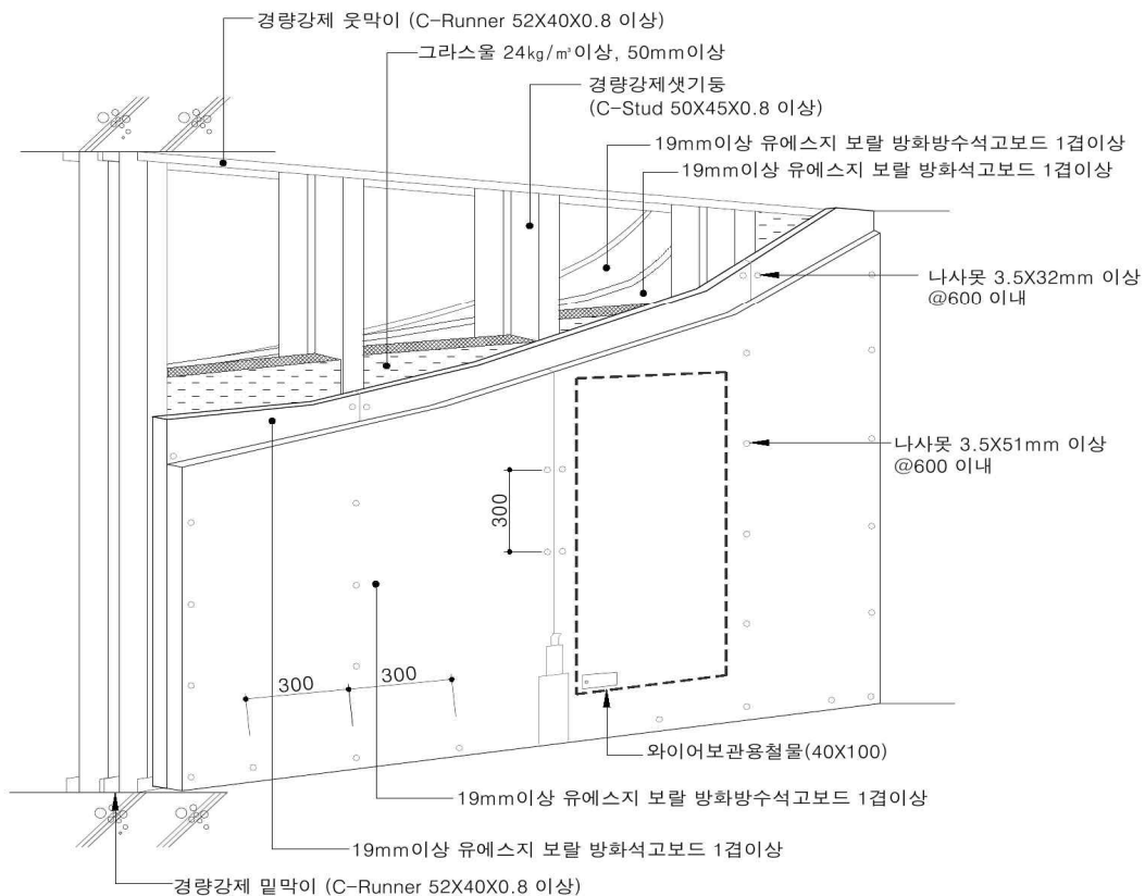
<투시도>
