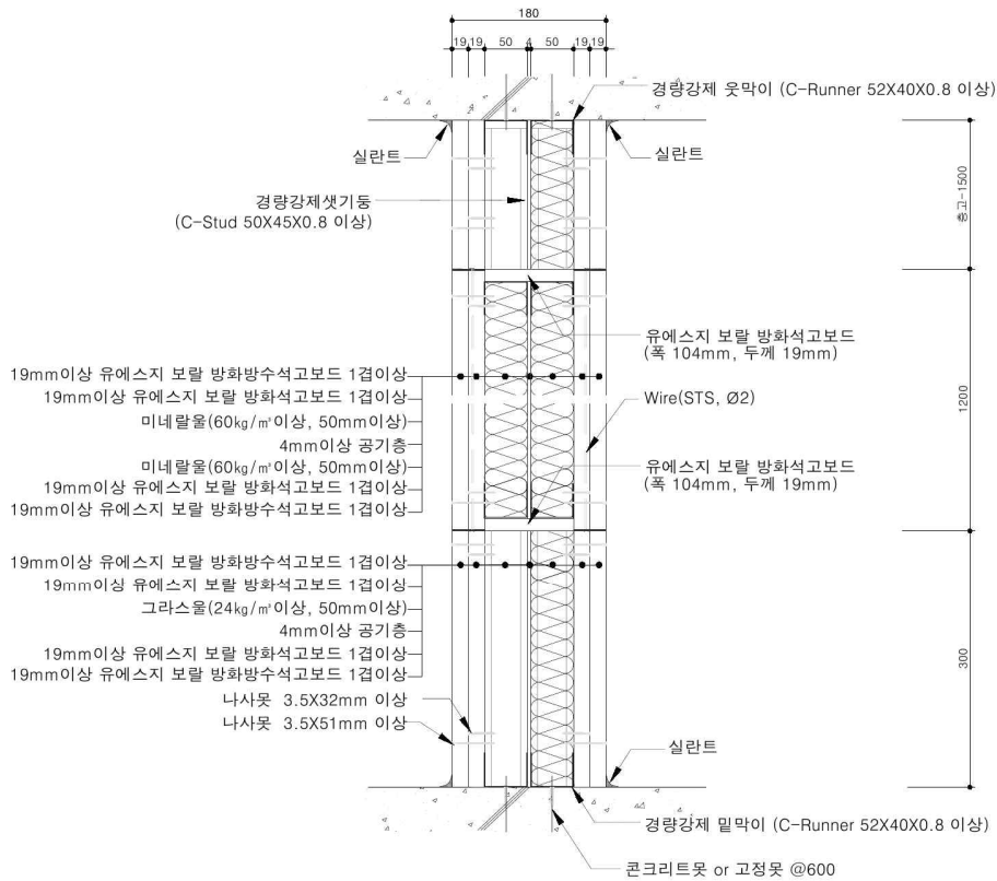
<수직단면도>
