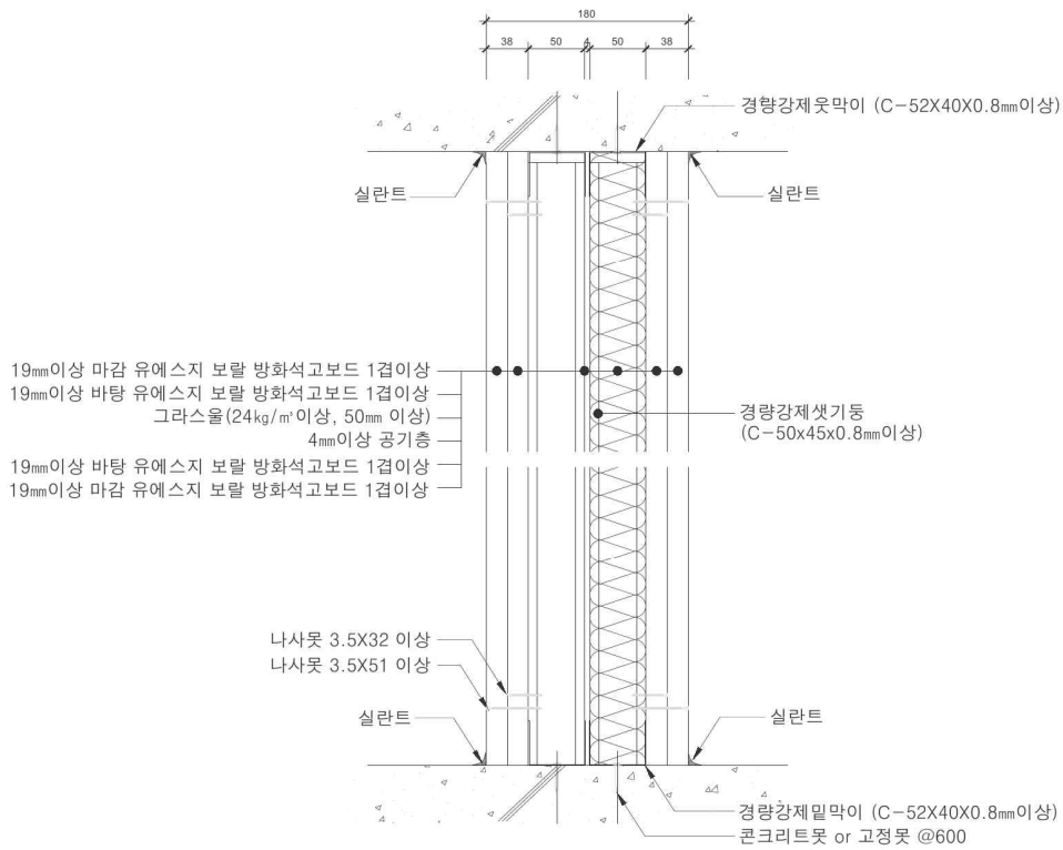
<수직 단면도>
