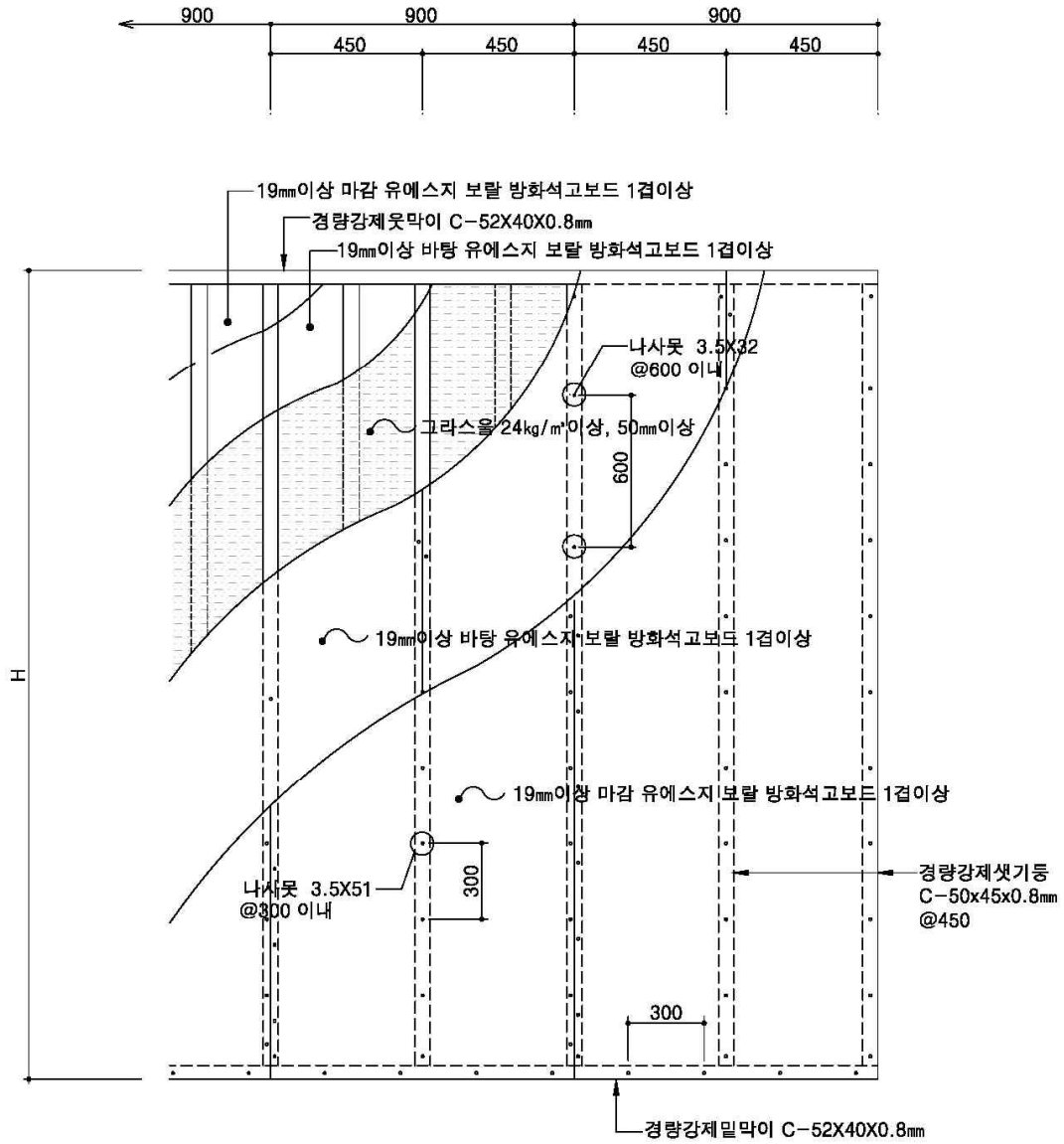
<입면도>
