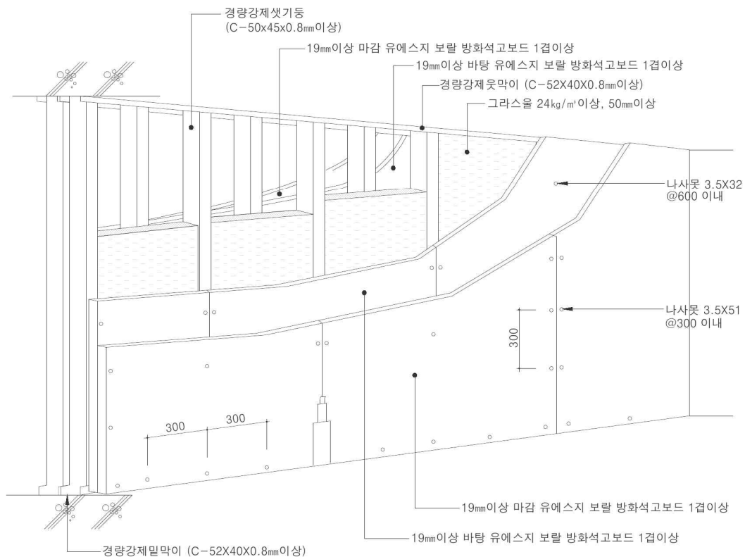
<투시도>
