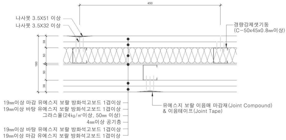
<수평 단면도>
