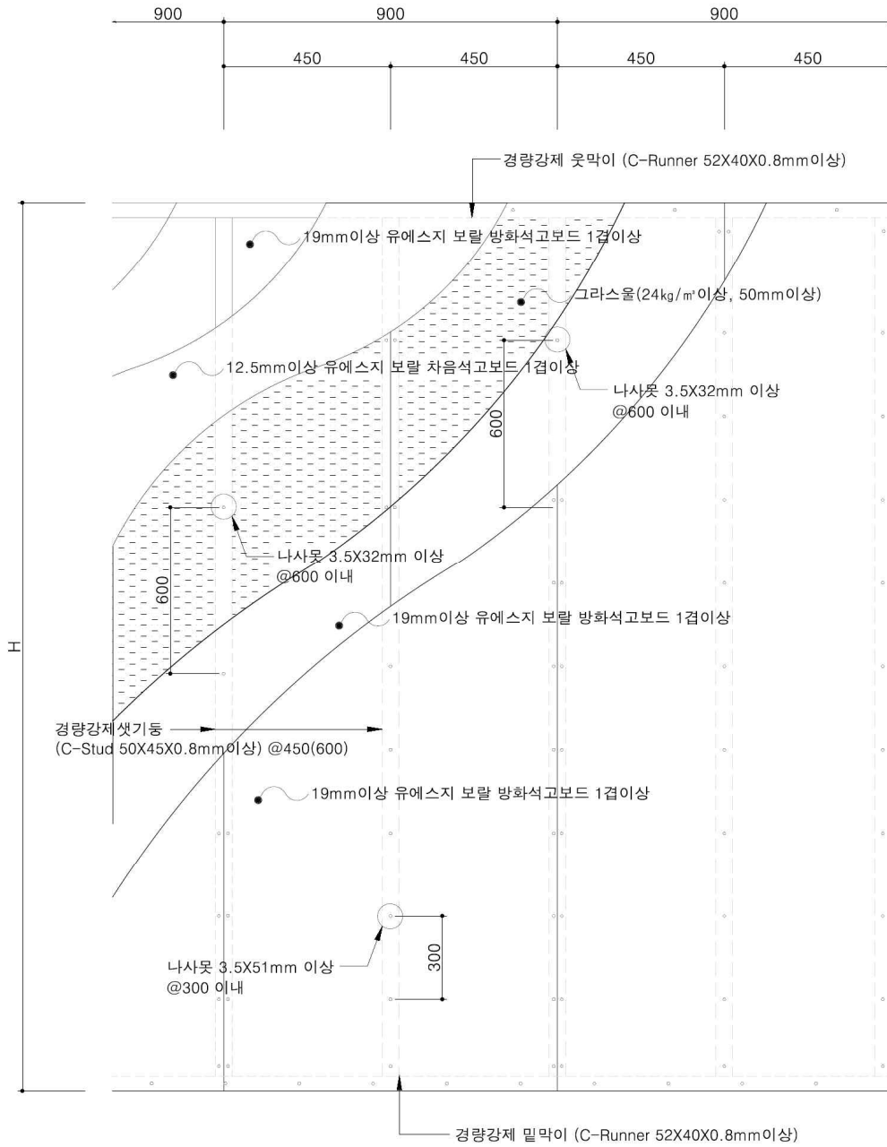
<입면도>
