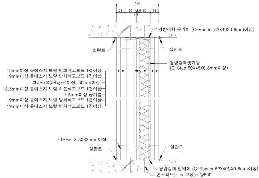
<수직단면도>
