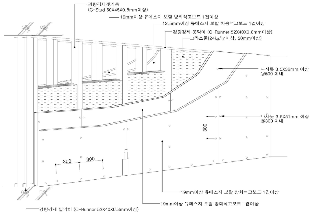
<투시도>
