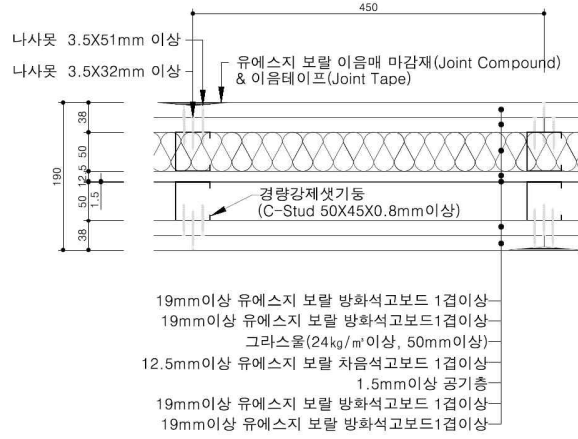
<수평단면도>
