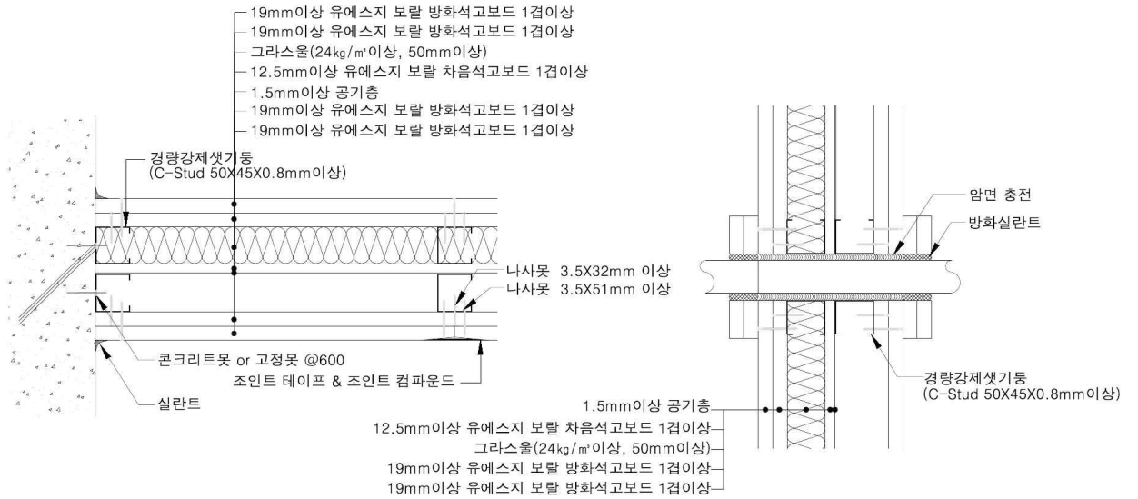
[ 벽 접합부위 상세도 ]
