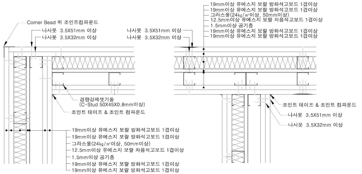
[ “ㄱ” 접합부위 상세도 ]
