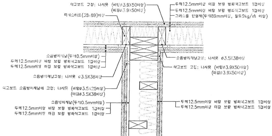
“T” 접합 상세도
