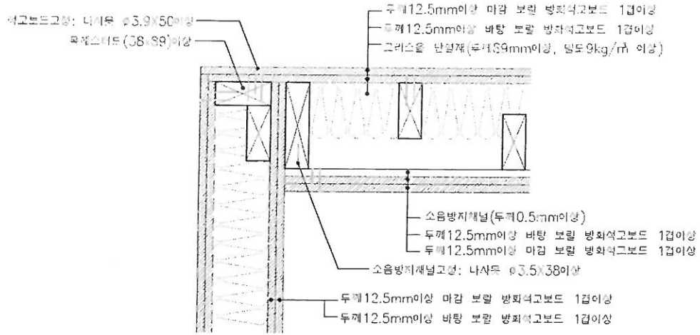
“ㄱ” 접합 상세도
