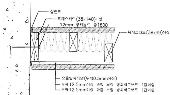
벽 접합 상세도
