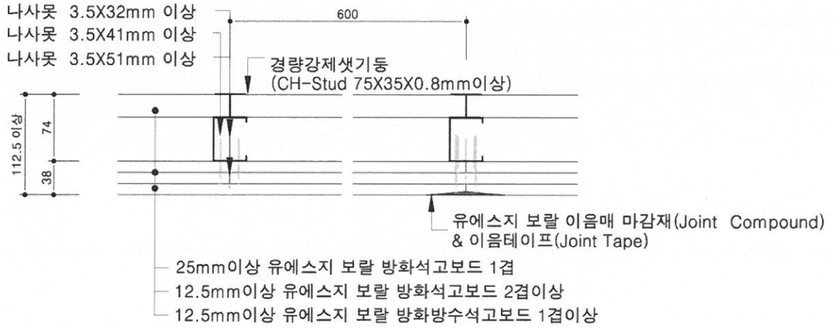
[수평단면 상세도]
