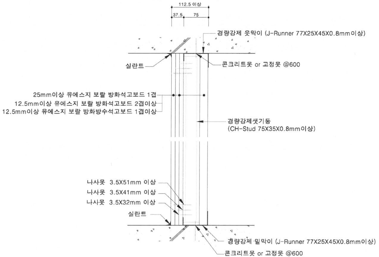
[수직단면 상세도]
