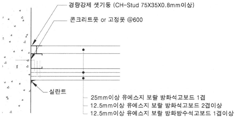
[ 벽 접합 상세도 ]
