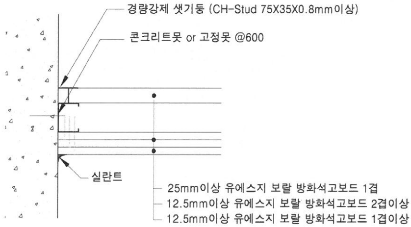
[ 벽 접합 상세도 ]
