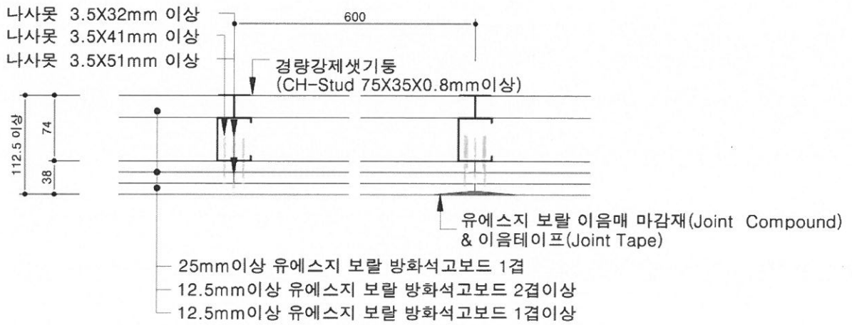
[수평단면 상세도]
