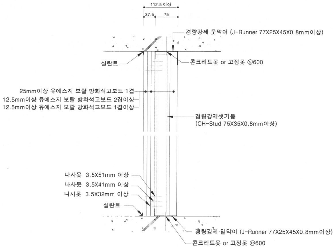
[수직단면 상세도]
