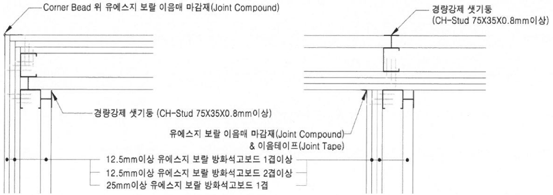
[ “ㄱ” / “T” 접합부위 상세도 ]
