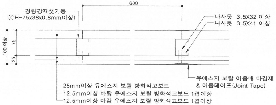
[수평단면 상세도]
