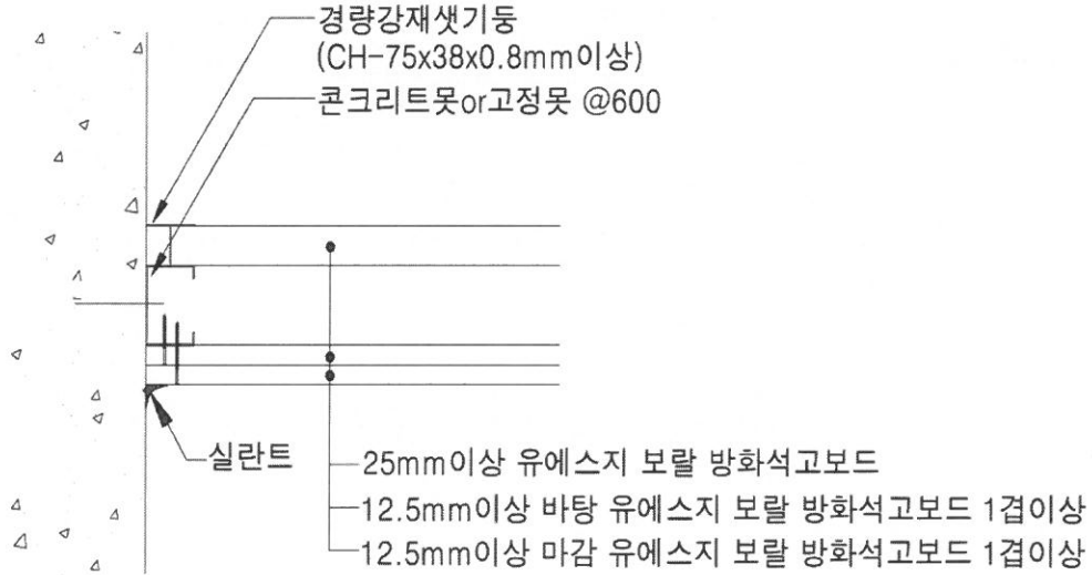
[ 벽 접합 상세도 ]
