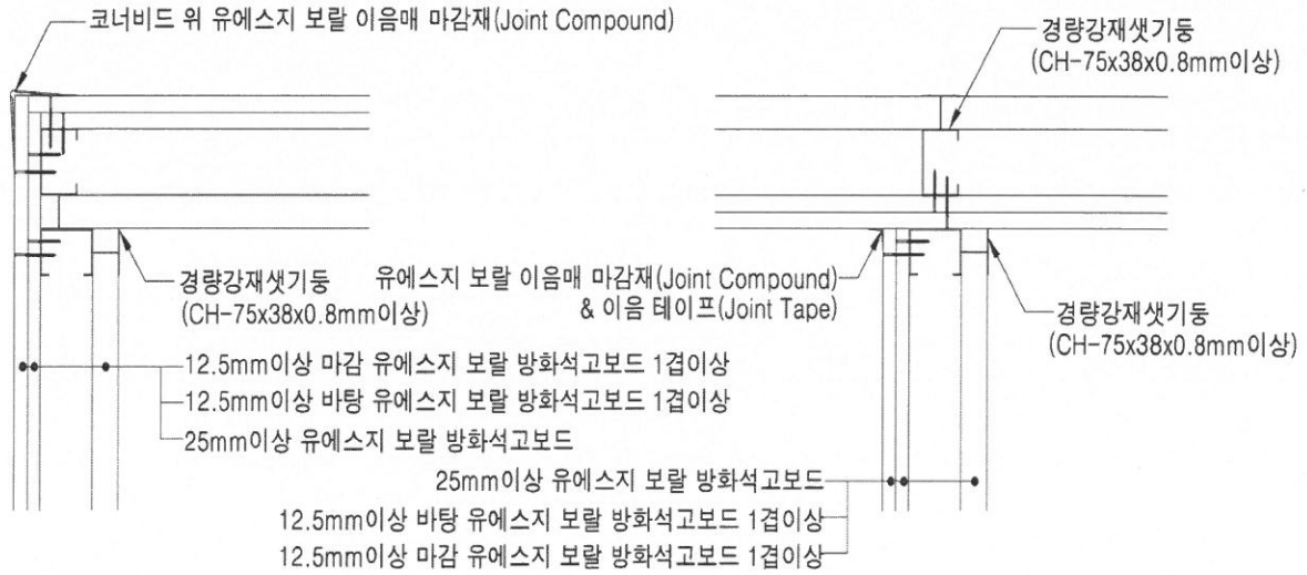
[ “ㄱ” / “T” 접합부위 상세도 ]
