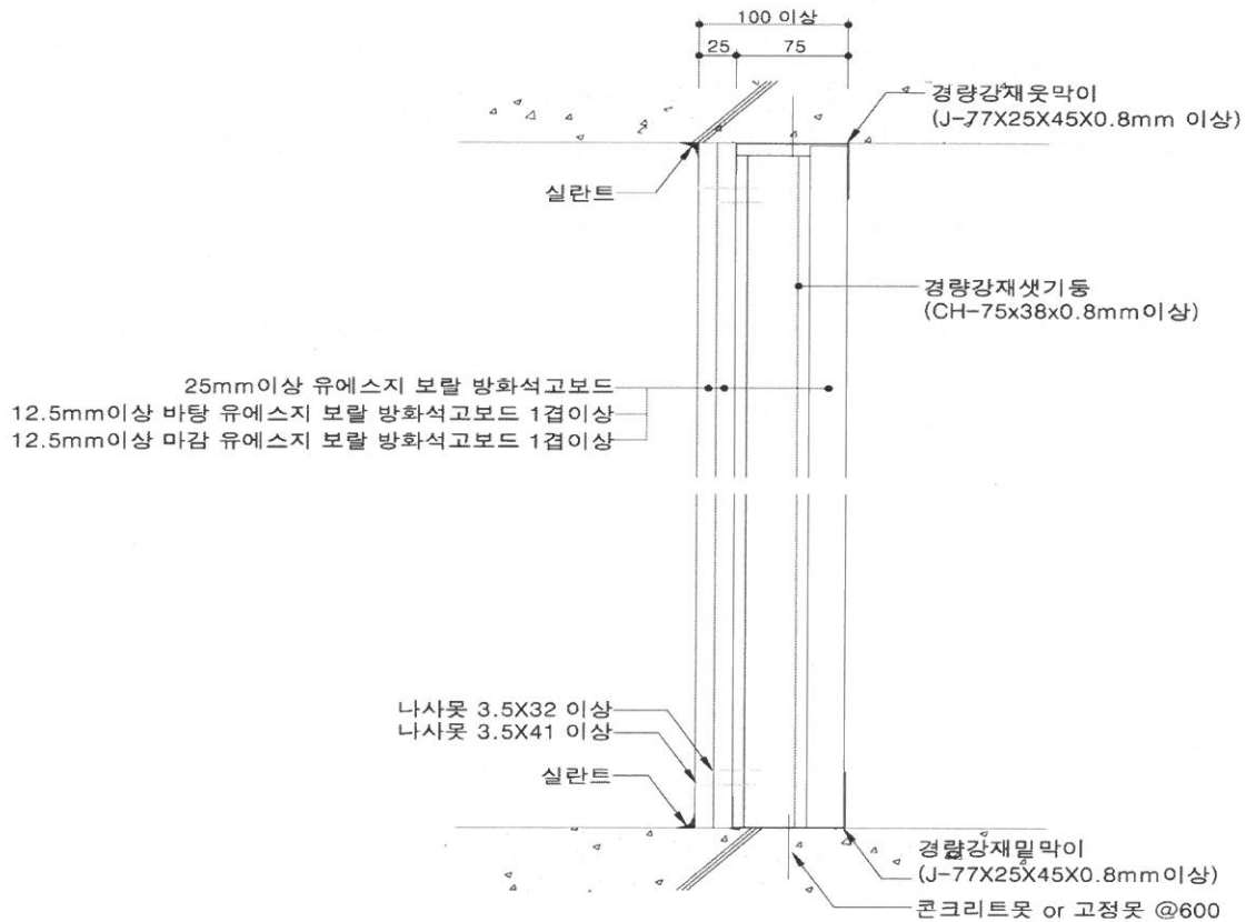
[수직단면 상세도]
