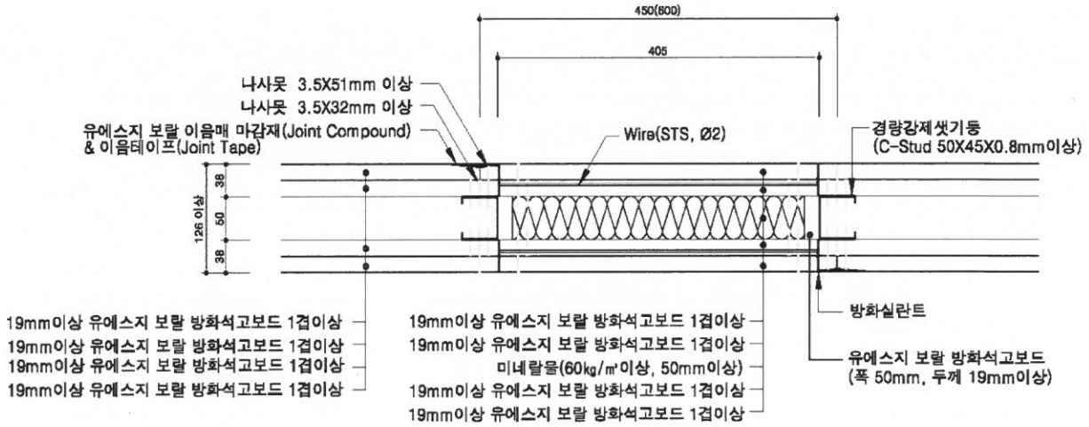
[수평단면 상세도]
