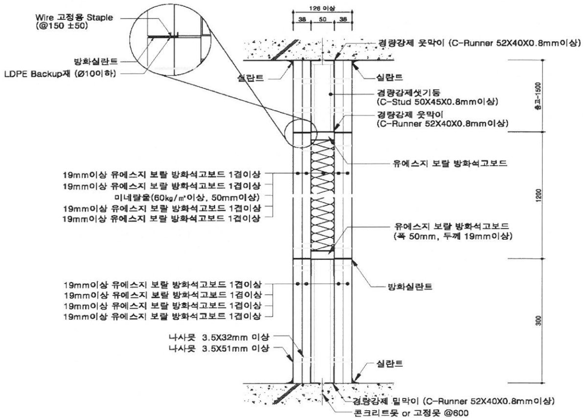
[수직단면 상세도]
