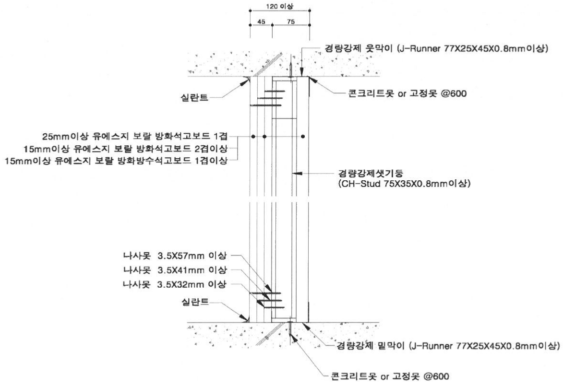
나. 수직 단면도
