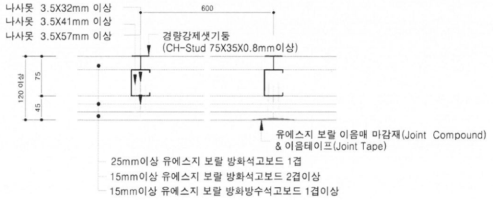
가. 수평 단면도
