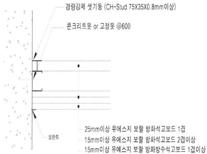
다. 벽 접합 상세도
