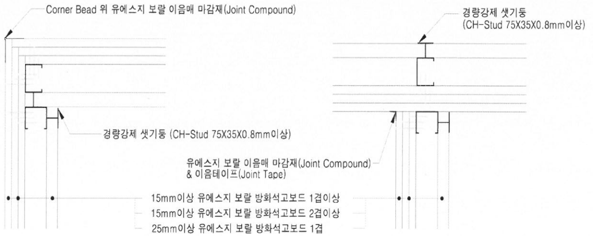
가. “L”접합상세도
