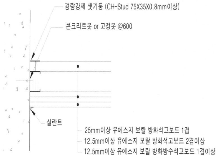
다. 벽 접합 상세도
