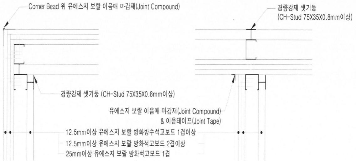
가. “┌”접합상세도
