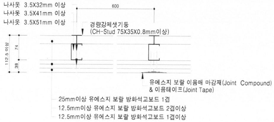
가. 수평 단면도
