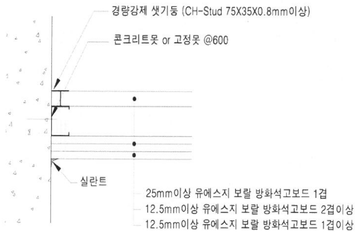
다. 벽 접합 상세도
