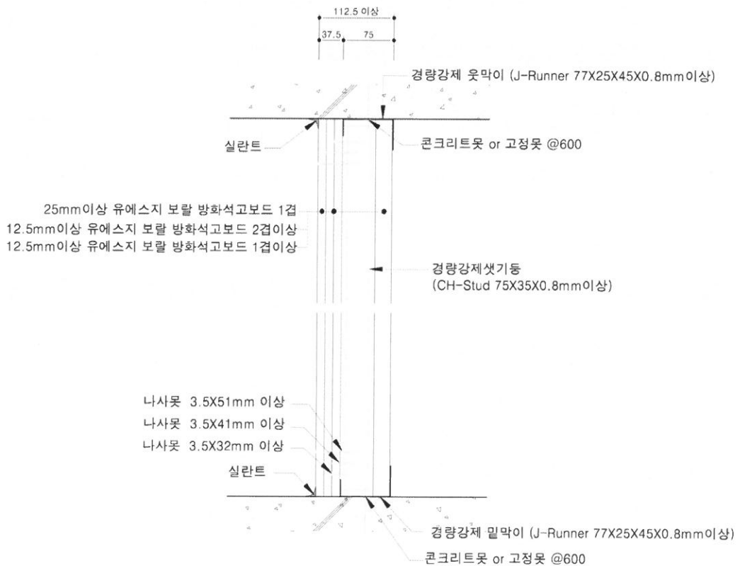
나. 수직 단면도
