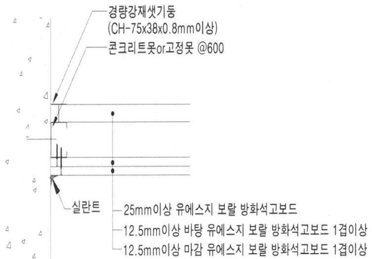
다. 벽 접합 상세도
