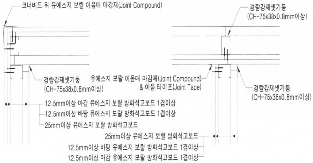
가. “G”접합상세도
