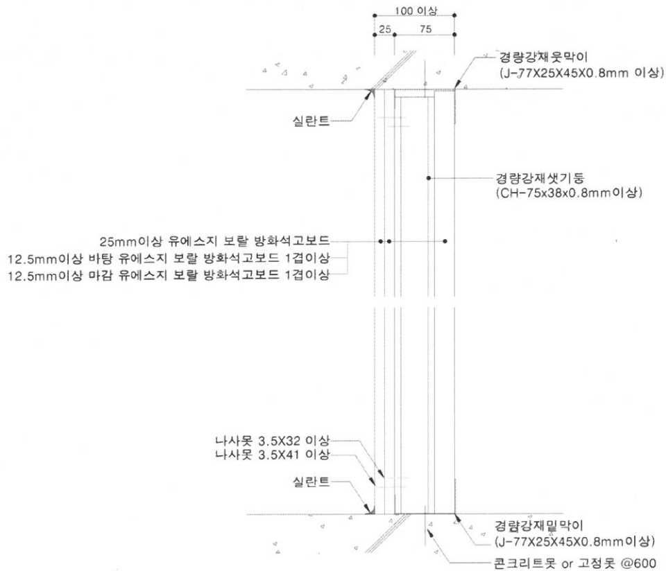
나. 수직 단면도
