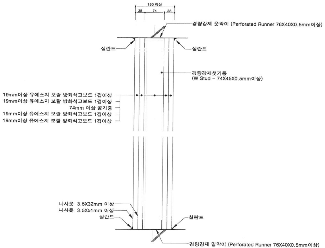
[수직단면 상세도]
