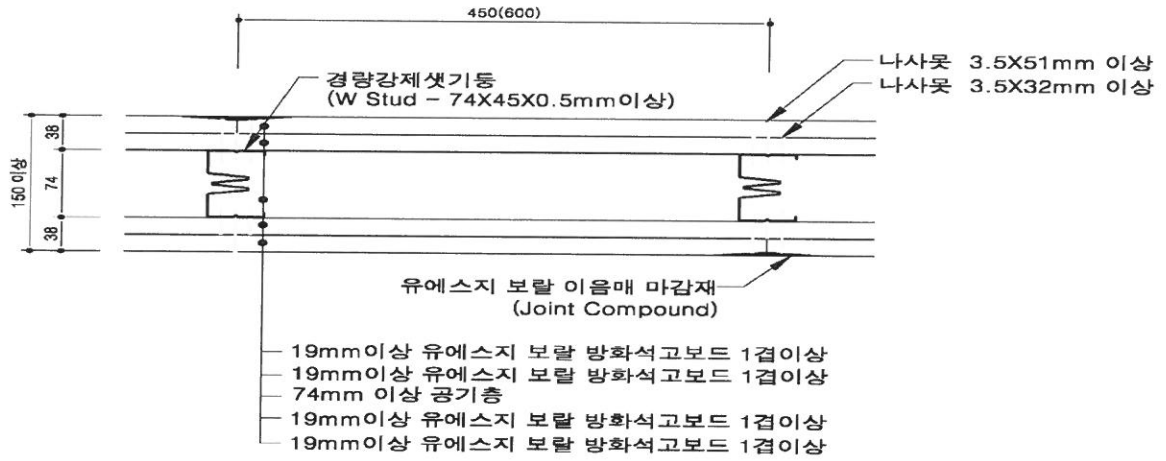
[수평단면 상세도]
