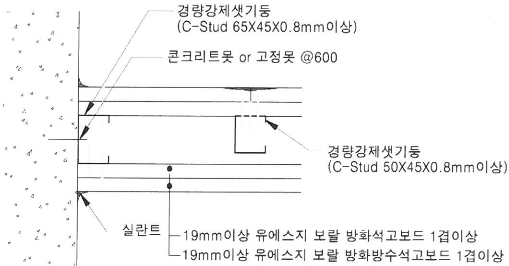
[ 벽 접합 상세도 ]
