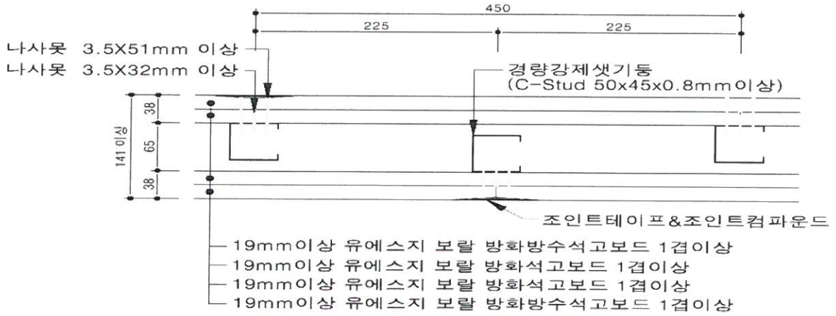
[수평단면 상세도]
