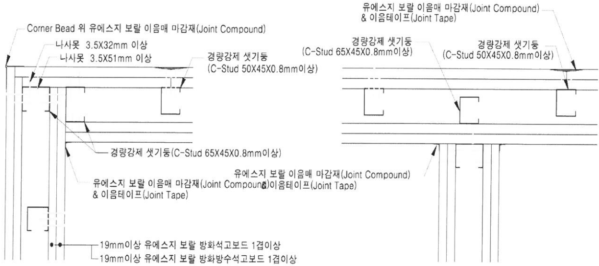
[ “ㄱ” / “T” 접합부위 상세도 ]
