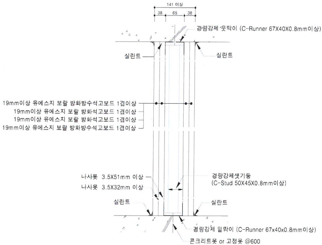
[수직단면 상세도]
