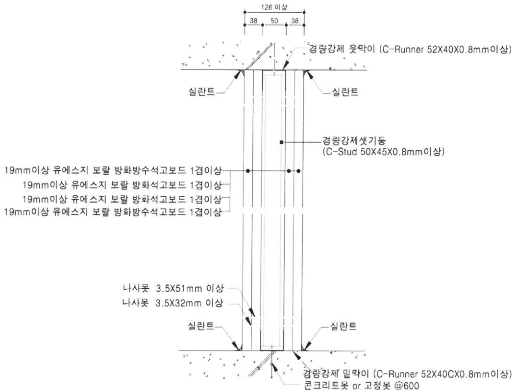
[수직단면 상세도]
