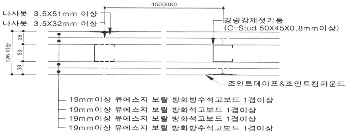
[수평단면 상세도]
