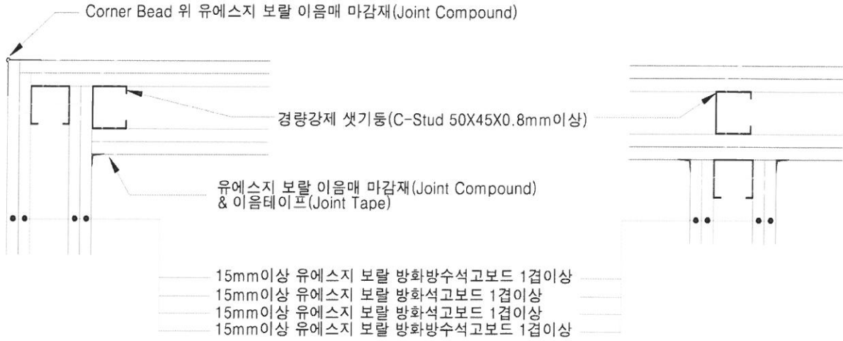
[ “┌” / “T” 접합부위 상세도 ]
