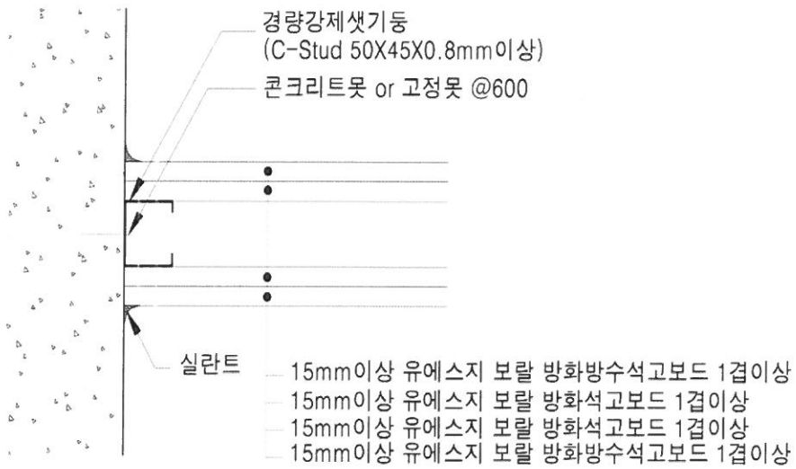
[ 벽 접합 상세도 ]
