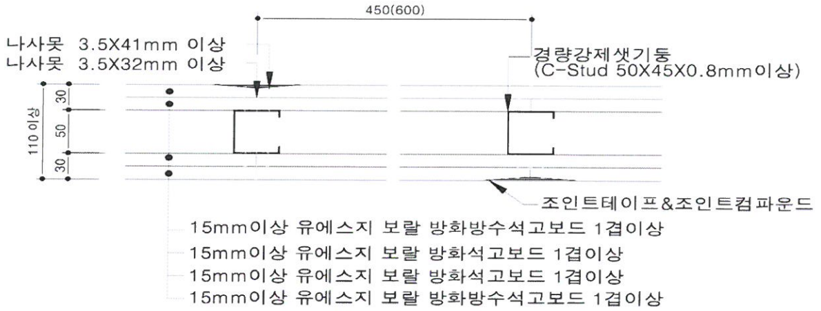
[수평단면 상세도]
