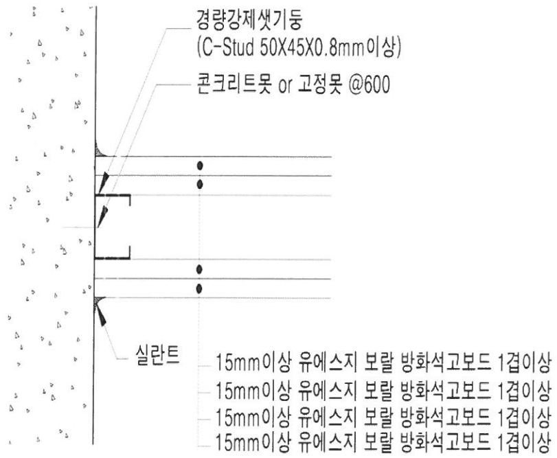
[ 벽 접합 상세도 ]
