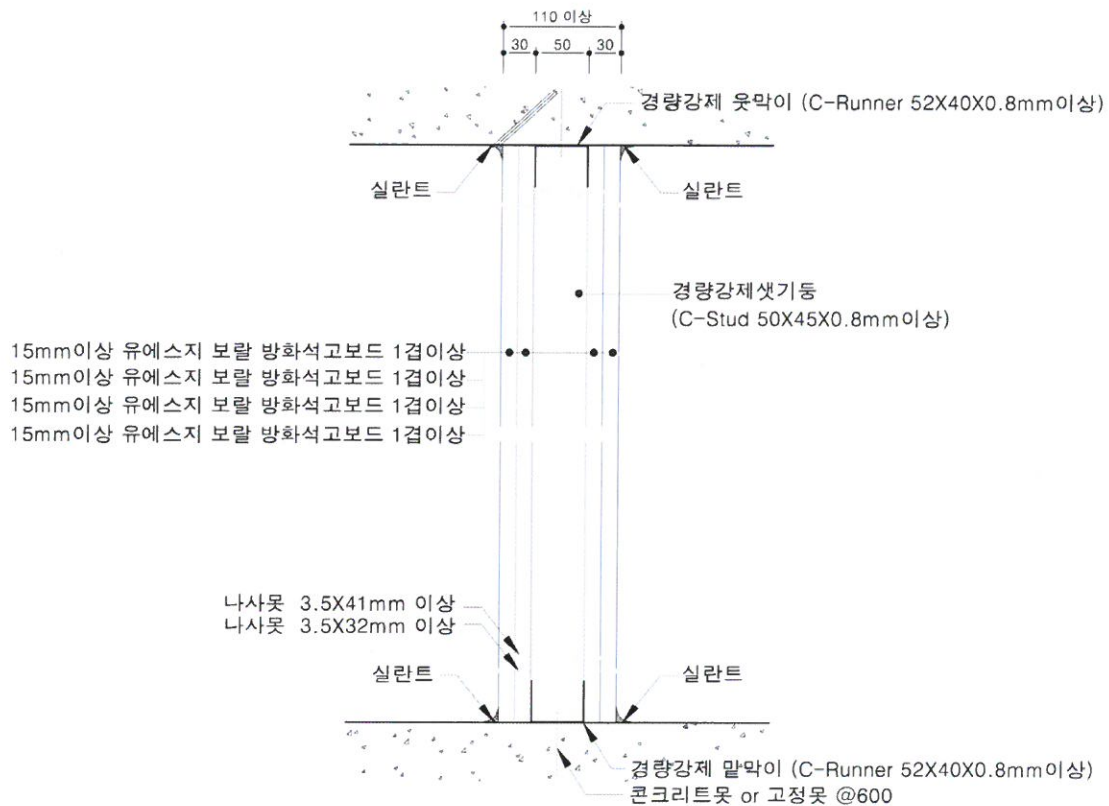
[수직단면 상세도]
