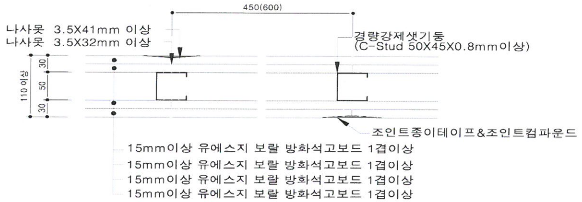
[수평단면 상세도]
