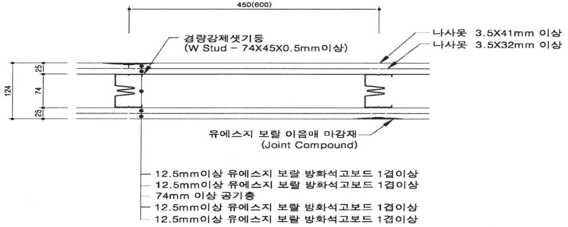
[수평단면 상세도]
