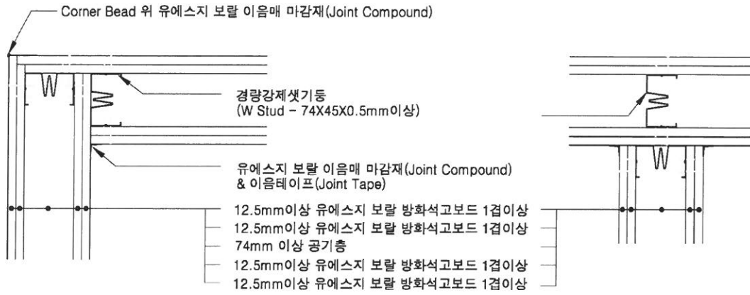
[ “ㄱ” / “T” 접합부위 상세도 ]
