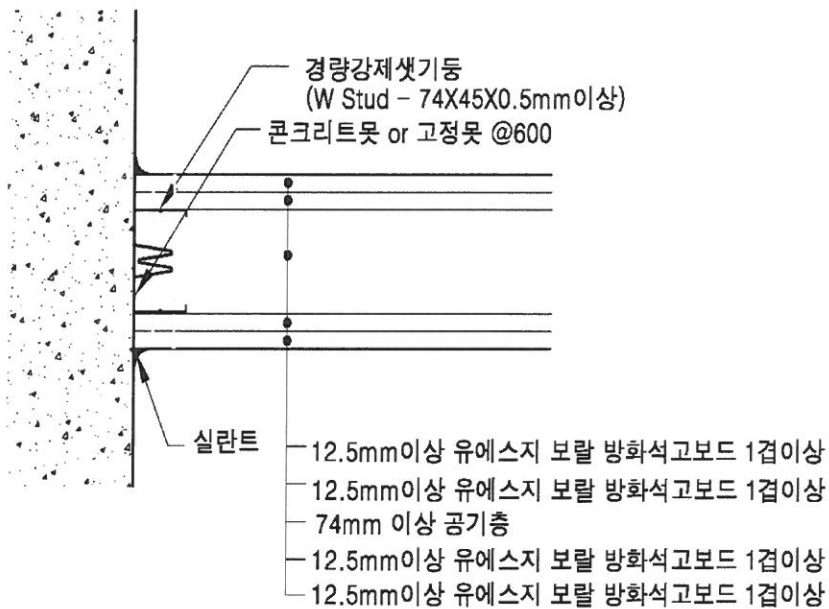
[ 벽 접합 상세도 ]
