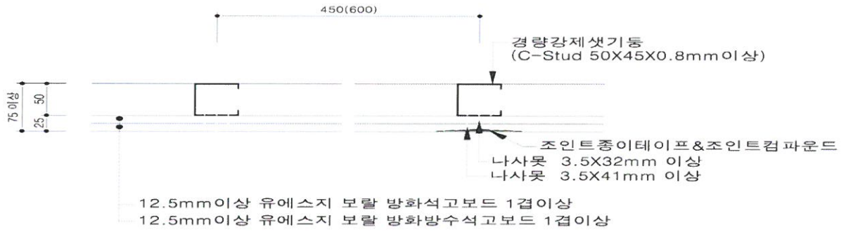
[수평단면 상세도]
