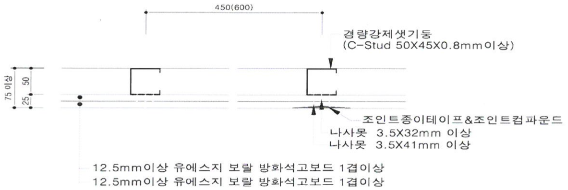
[수평단면 상세도]
