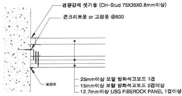
[벽 접합 상세도]
