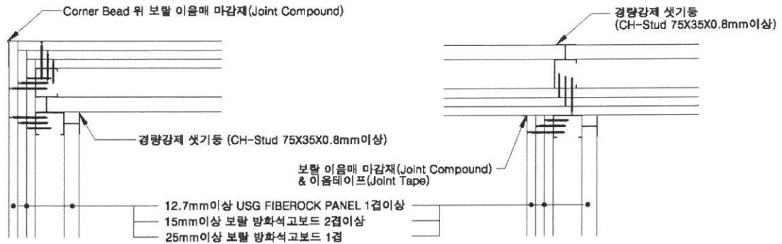
[“T” 접합부 기준 상세]
