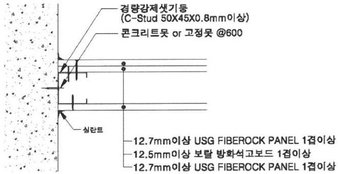
[벽 접합 상세도]
